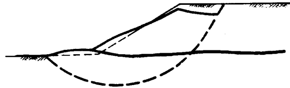
Fig. 12.5. ROTURA CIRCULAR CORTANDO EL REFUERZO
