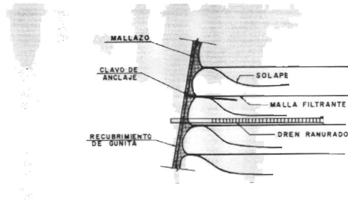
Fig. 13.5. ACABADO DE PARAMENTOS Y DRENAJE
