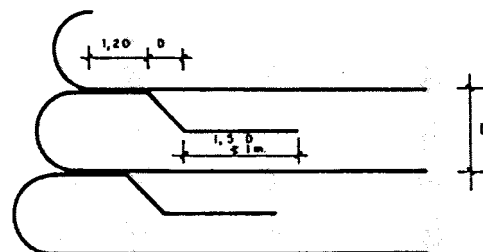
Fig. 13.2. CONFIGURACIÓN DEL MACHON DE ANCLAJE
