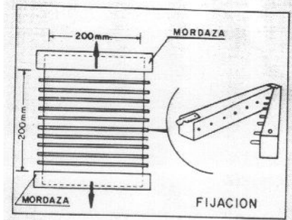
b) ENSAYO DE TRACCION CON FIJACIONES
