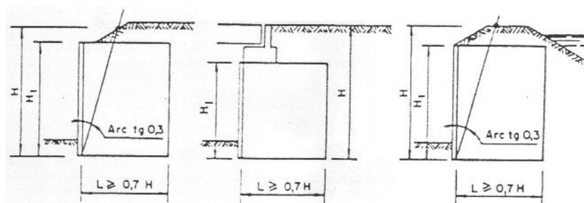
Fig. 6.5. GEOMETRIA DE LAS SECCIONES TRANSVERSALES
