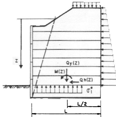
Fig. 7.6. DETERMINACION DE LA TENSION \sigma_1 EN UN MURO
