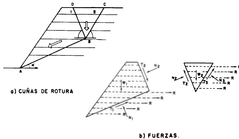
Fig. 12.10. EQUILIBRIO DE UN MECANISMO DE DOBLE CUÑA
