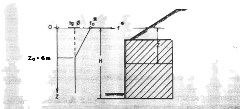
Fig. 5.5. DETERMINACION DE f^* EN FUNCION DE LA PROFUNDIDAD
