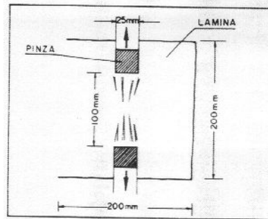
c) ENSAYO DE TRACCION CON PINZAS
