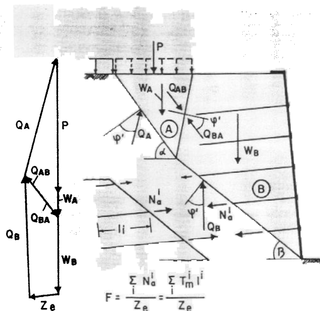
Fig. 9.6. ESQUEMA DE COMPROBACION DE LA ESTABILIDAD DE UNA CUÑA DE SUELO COSIDO
