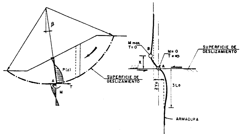
Fig. 9.3. COMPORTAMIENTO MECANICO DE UNA ARMADURA
