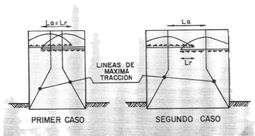
Fig. 7.12. LINEAS DE TRACCION MAXIMA Y LONGITUD DE ADHERENCIA EN LOS MUROS DOBLES
