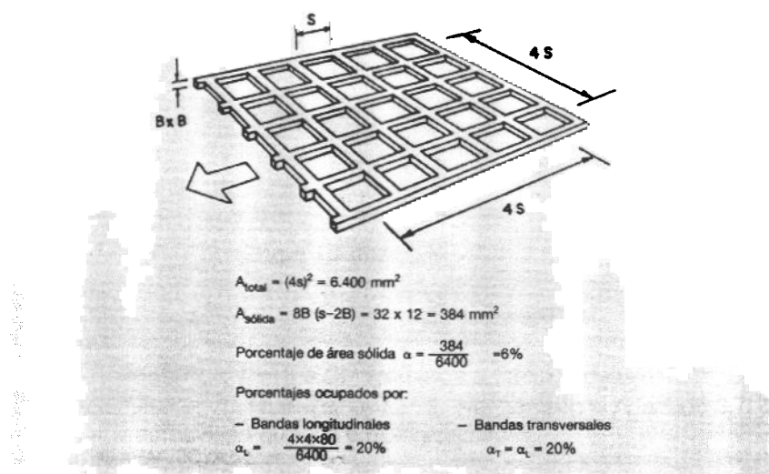
Fig. 11.2. DEFINICION DE AREA EFECTIVA
