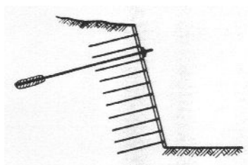
e) COSIDO Y ANCLAJE DE EXCAVACIONES SUBVERTICALES
