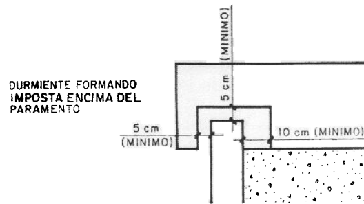
Fig. 8.7. UNION DEL DURMIENTE CON EL PARAMENTO
