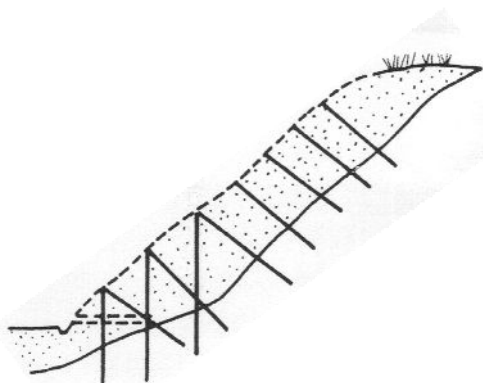
a) COSIDO DE UN MANTO COLUVIAL.
