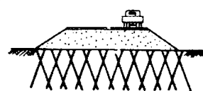
b) MEJORA DE LA ESTABILIDAD DE UN TALUD EN TERRENO BLANDO.
