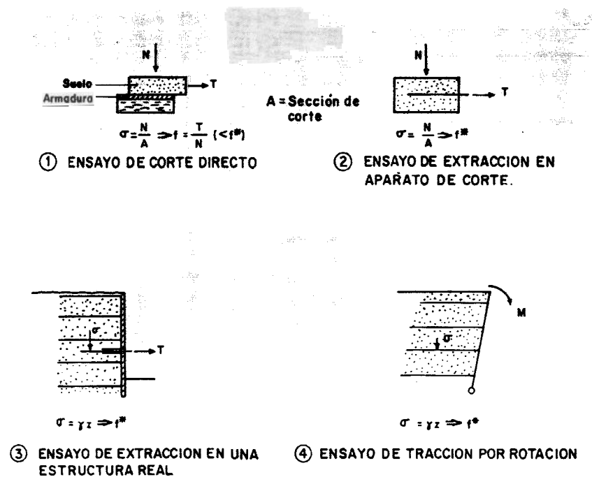
Fig. 5.1. ENSAYOS PARA LA DETERMINACION DEL ROZAMIENTO SUELO-ARMADURA
