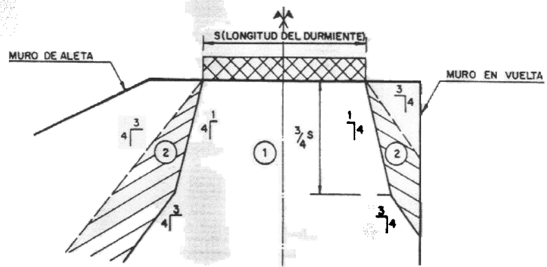
Fig. 7.8. DIFUSION PARALELA A LA LINEA DE APOYO
