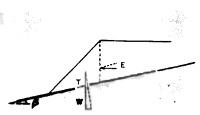
Fig. 12.4. CASC DE TERRAPLEN SOBRE CIMIENTO INCLINADO
