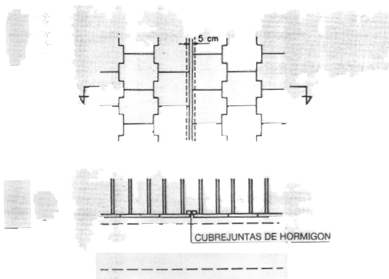
Fig. 5.7. JUNTAS VERTICALES EN LOS PARAMENTOS DE PLACAS DE HORMIGON
