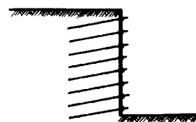
e) COSIDO Y ANCLAJE DE EXCAVACIONES SUBVERTICALES
