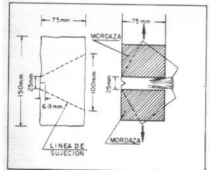
d) ENSAYO DE DESGARRAMIENTO
